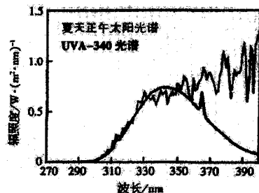
图1 UVA-340光谱与夏天正午太阳光谱比较
