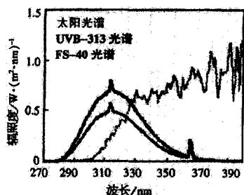
图2 UVB-313及FS-40光谱与太阳光谱比较
